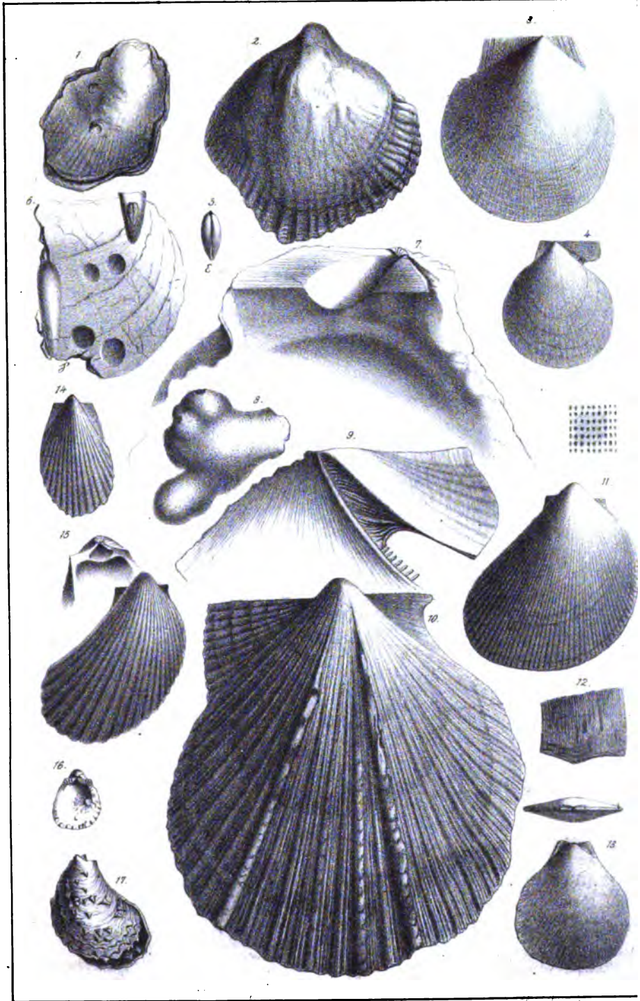
Quenstedt Jura.
